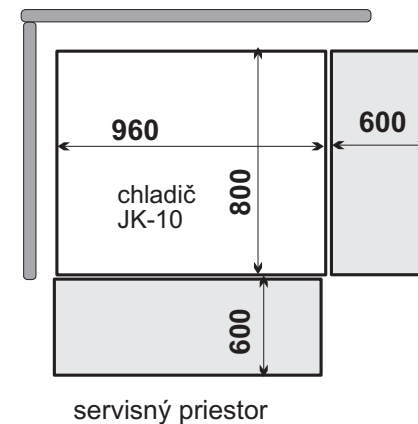
UMIESTNENIE CHLADIČA
