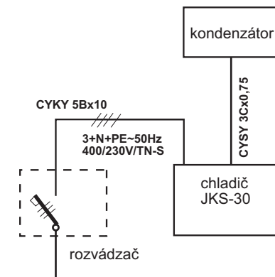
ELEKTRICKÉ PRIPOJENIE
